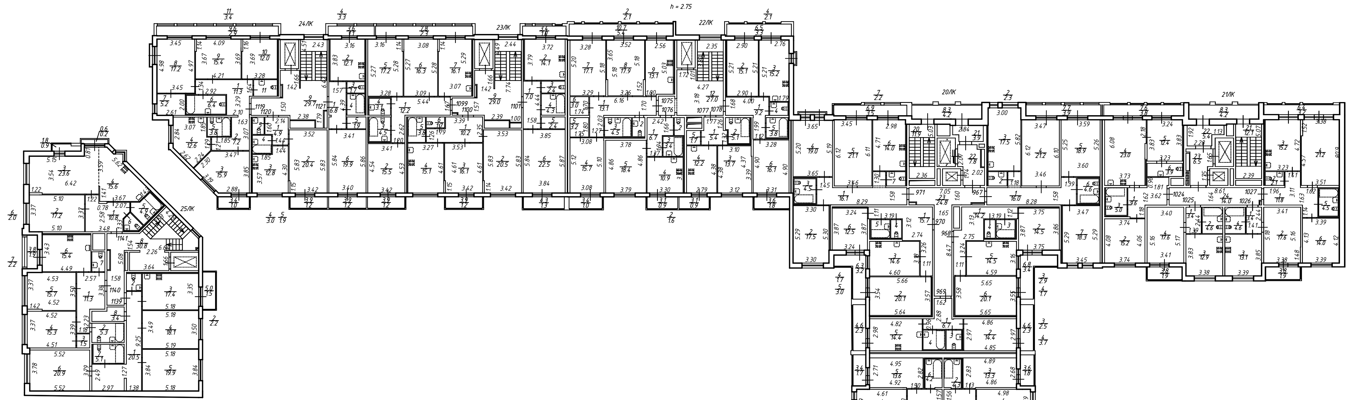
План 5 этажа
